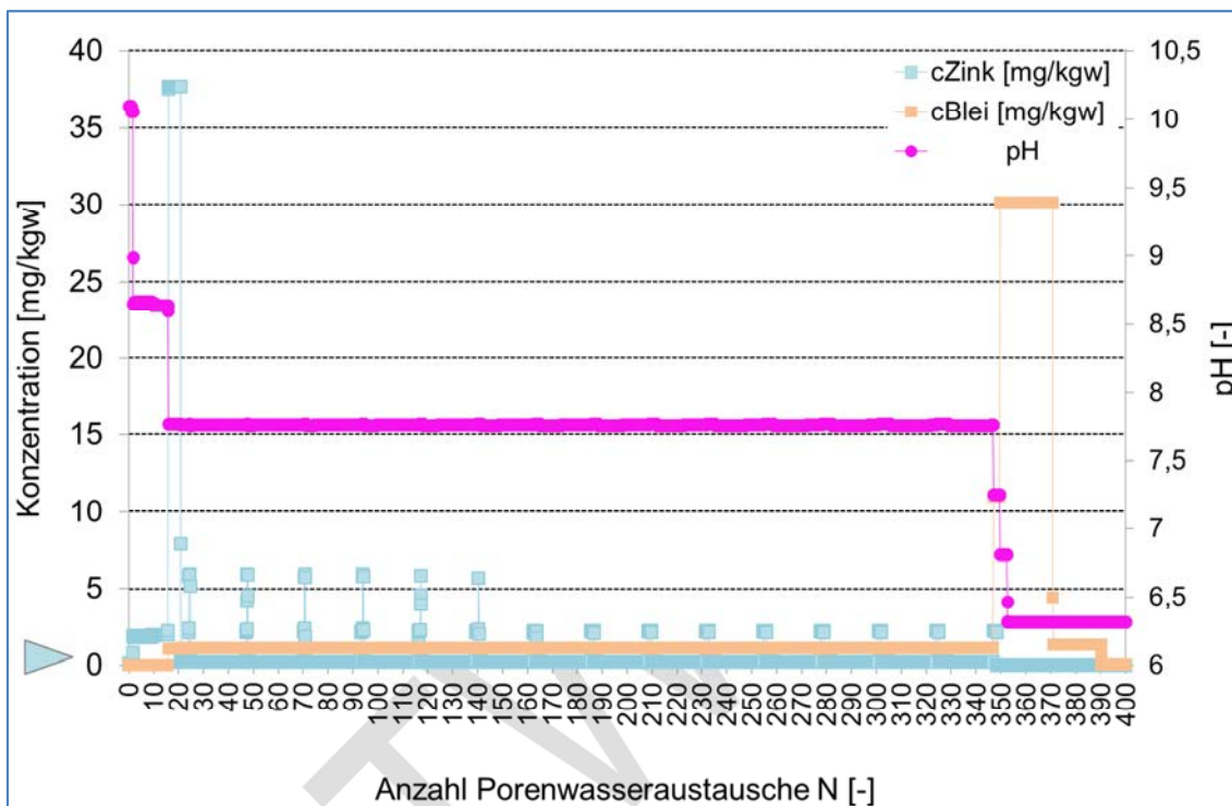
Abb. 28: Standardszenario: Entwicklung der pH-Werte sowie der Zink- und Bleikonzentrationen in den Porenwässern der letzten (der 15.) Reaktorzelle (mg/kgw entspricht näherungsweise mg/L) [REDACTED]
