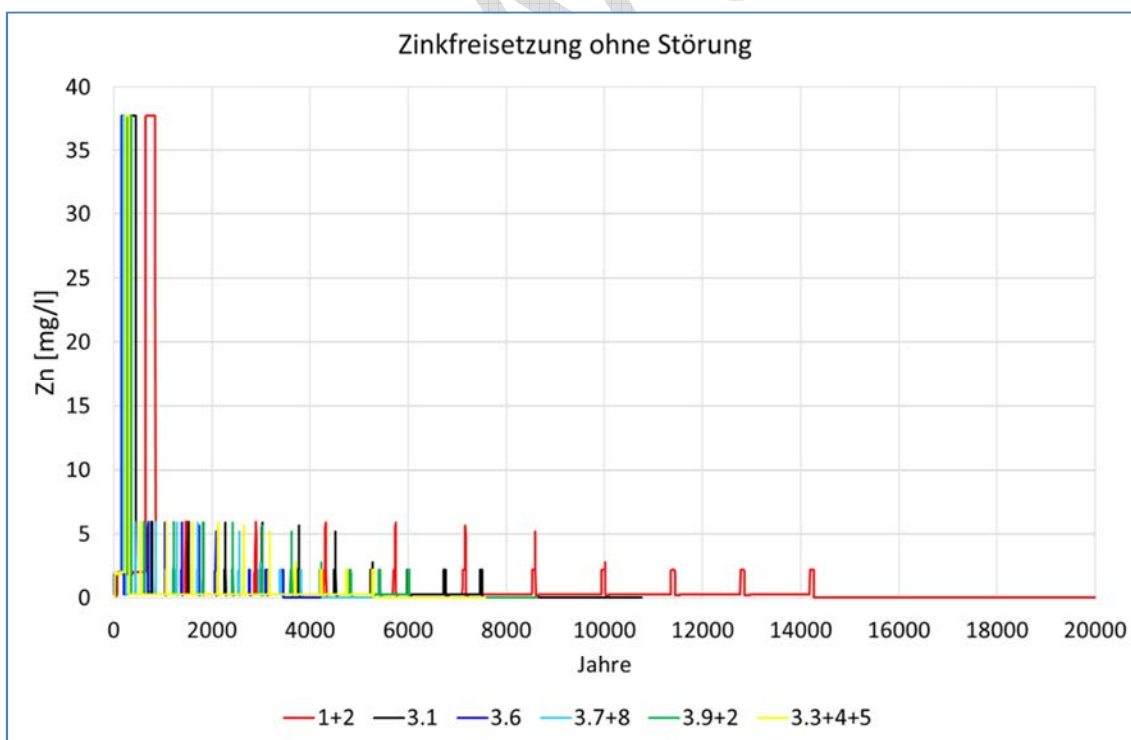
Abb. 49: Beginn und Dauer der Freisetzung von Zink aus den BHV-Bereichen bei einer Fließlänge von 15 m und 10 % Reststoffen im Reaktionskontakt (Quellterm) (Quelle: delta h)
