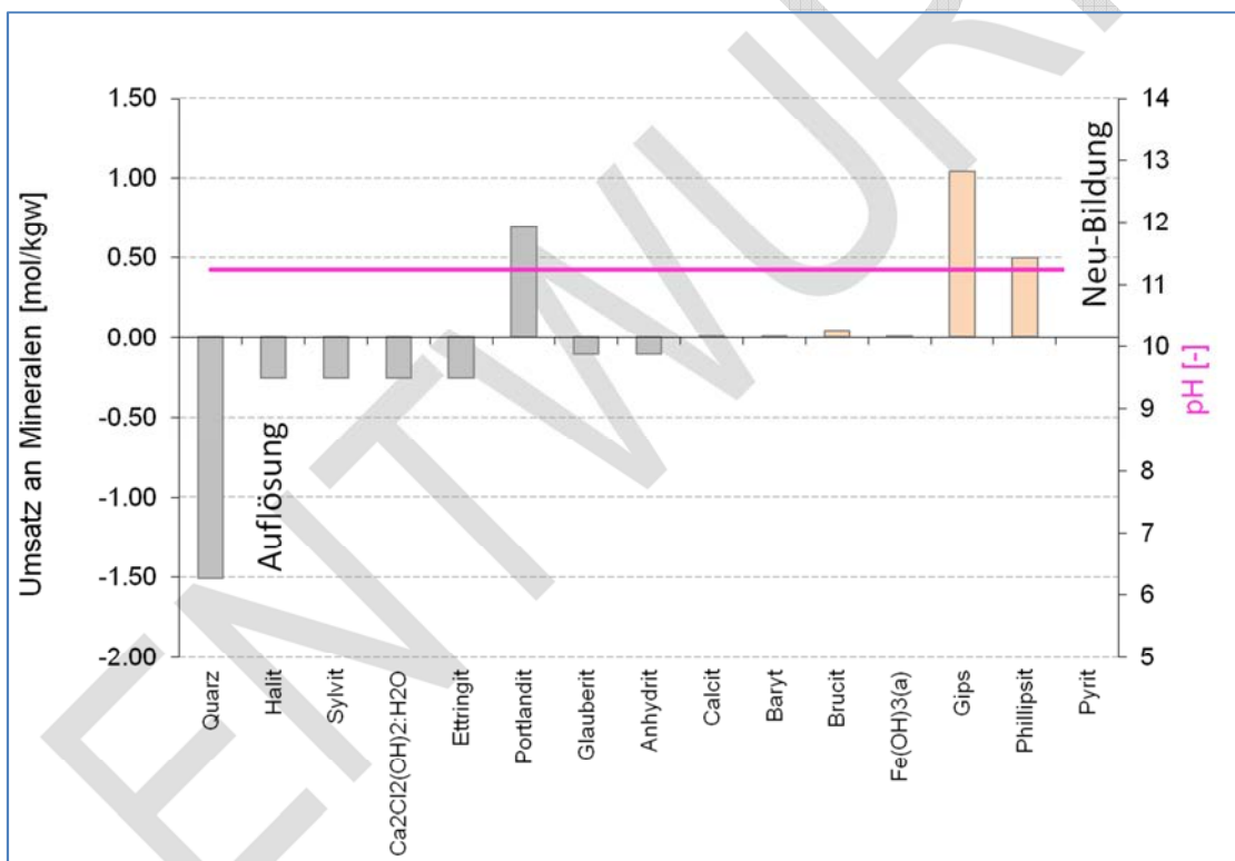
Abb. 26: Auflösung und Neubildung von Mineralphasen in 1 L Tiefengrundwasser bei einem sich dabei einstellenden pH-Wert von ca. 11,5 ( [REDACTED] )
