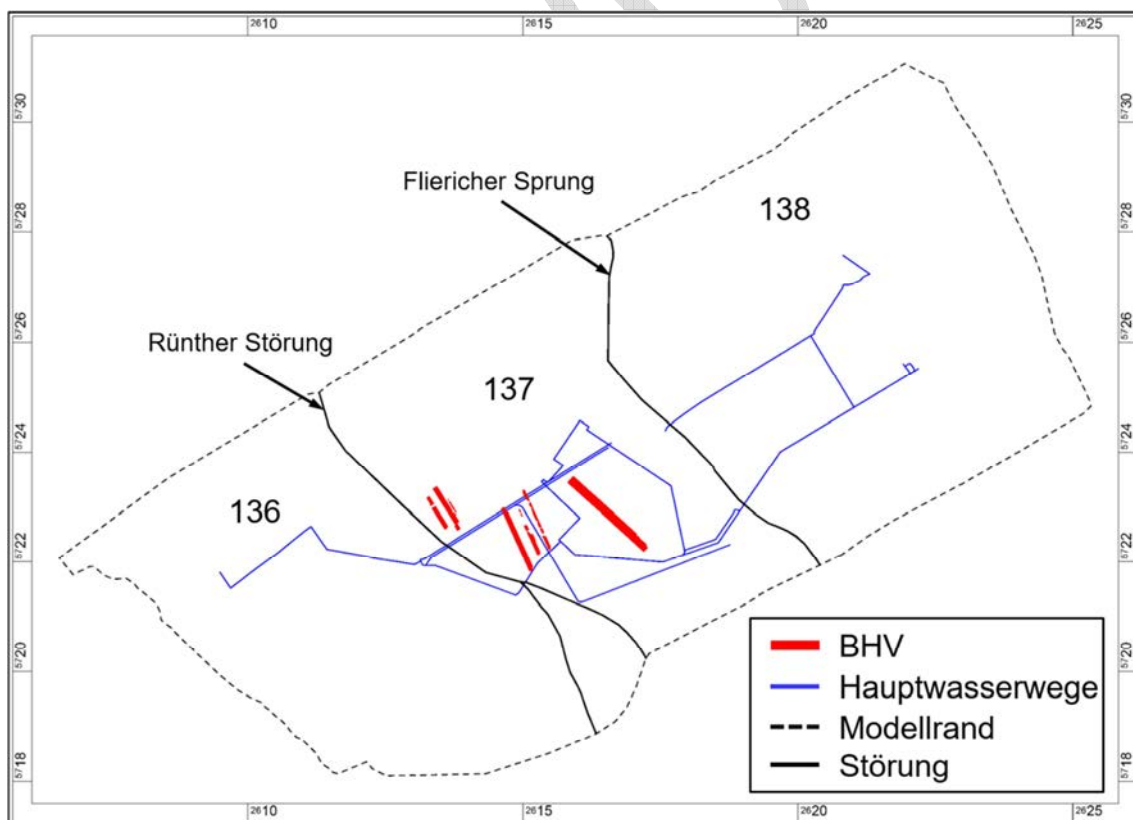
Abb. 32: Gesamtes Modellgebiet: Geologische Schollen, Hauptwasserwege (blau), Bruchhohlraumverbringung (rot), Modellrand (unterbrochene schwarze Linie), Störungen (schwarz), Schollennummern (Quelle: delta h)
