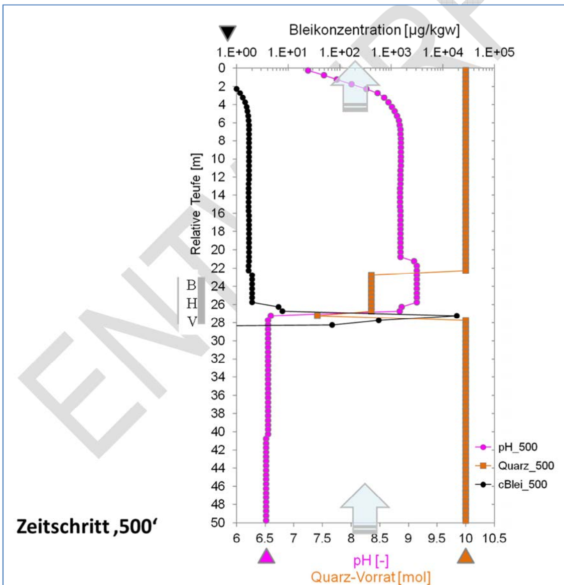
Abb. 27: Beispiel für eine 1D-Stofftransportmodellierung (Vorstudie) mit dimensionslosem Zeitschritt
