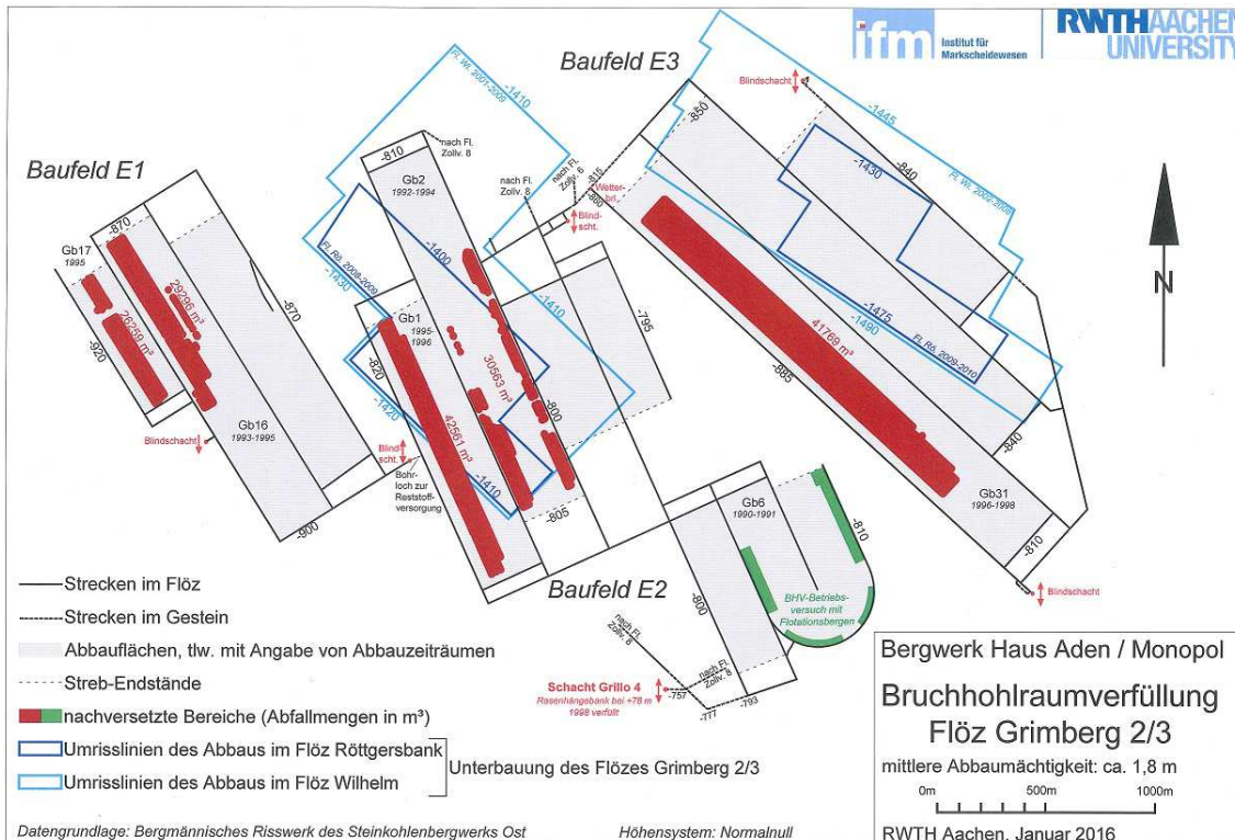
Abb. 9: Lage der Bauhöhen und Bereiche mit Bruchhohlraumverfüllung im Flöz Grimberg 2/3, Baufelder E1, E2 und E3 des BW Haus Aden/Monopol
