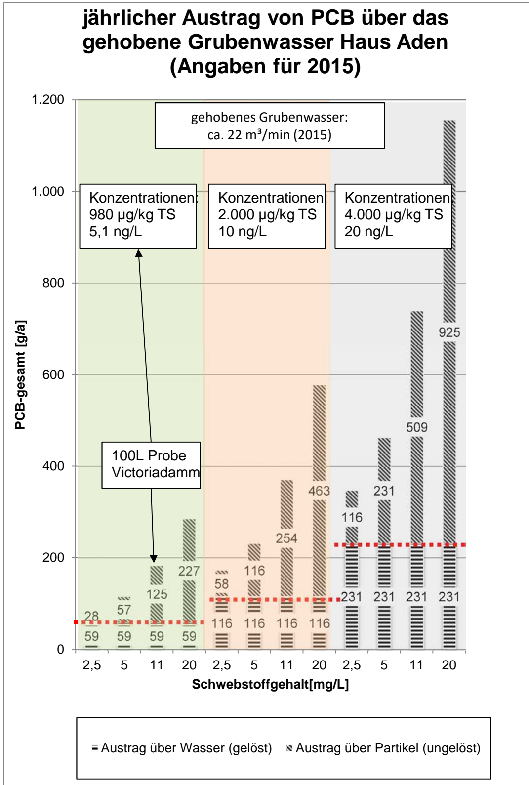
Abb. 67: Ergebnisse der 100-L-Grubenwasserprobe und Szenarios für jährliche Aus-tragsmengen bei sich ändernden Schwebstoffgehalten und PCB-Konzentrationen (wässrige Phase und partikulär-gebunden)
