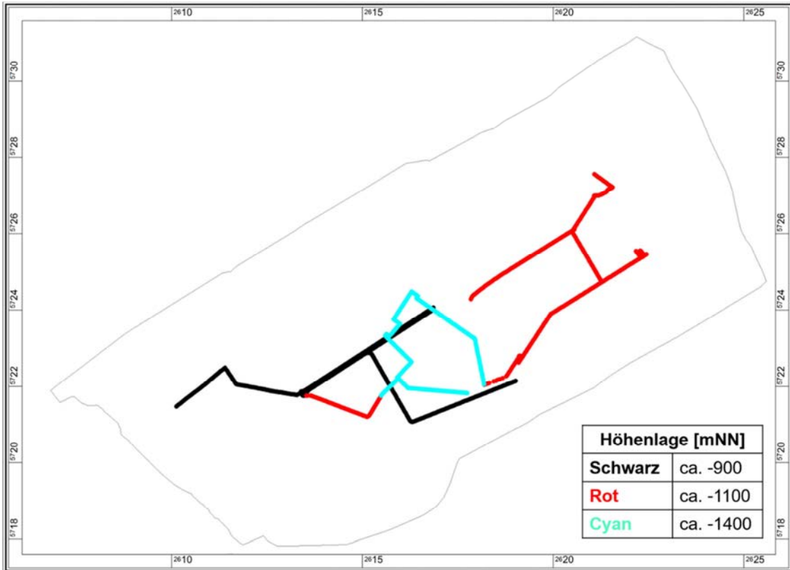
Abb. 39: Drainierende Modellknoten (Vorflutwirkung) im Röhrensystem ohne Störung (Quelle: delta)
