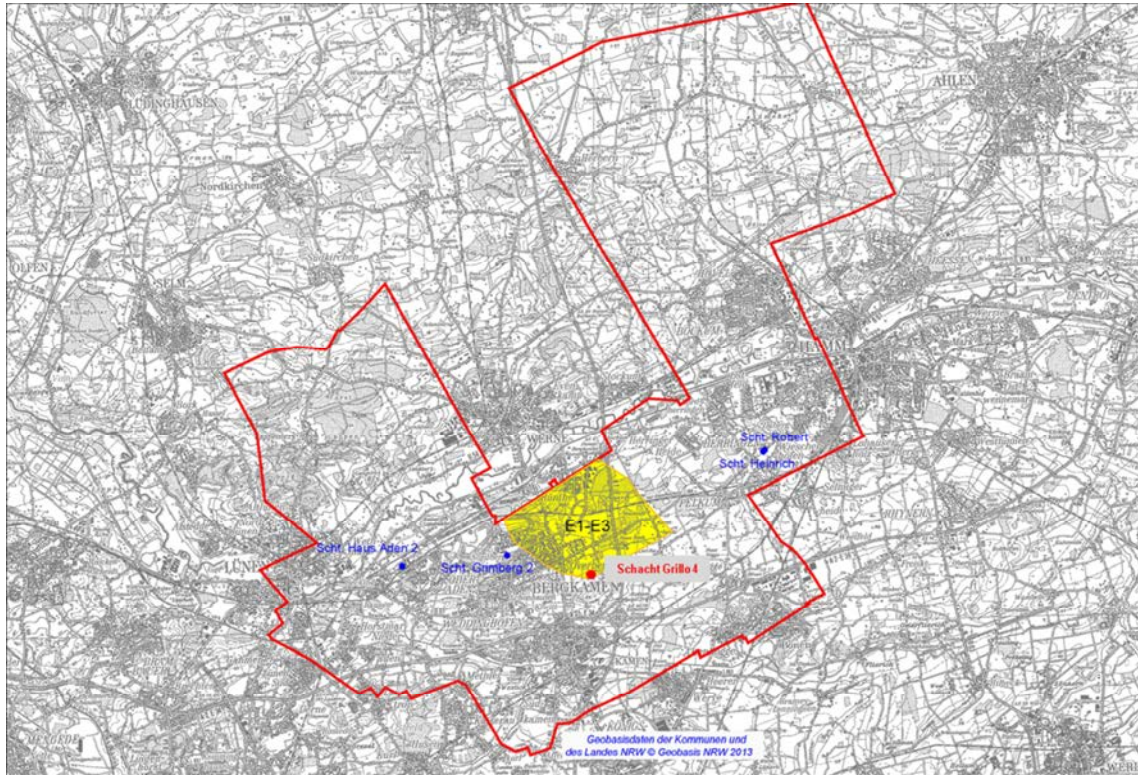
Abb. 6: Feldesgrenzen des Verbundbergwerks Ost (rot), Lage der Baufelder Monopol E1, E2, E3 (gelb), offen gehaltene Tagesschächte und Standort Schacht Grillo 4
